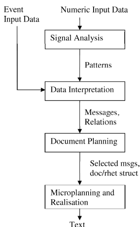
图 4.1: 数据到文本的生成系统的一般框架 [77]
